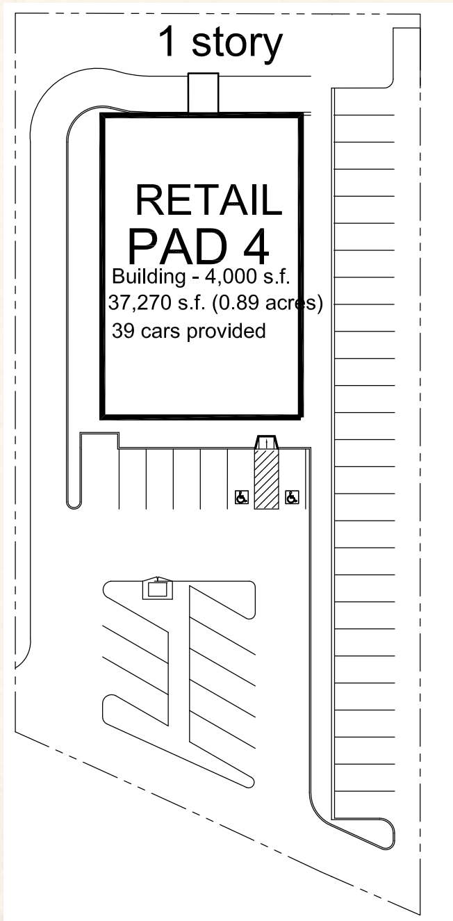
Siteplan
