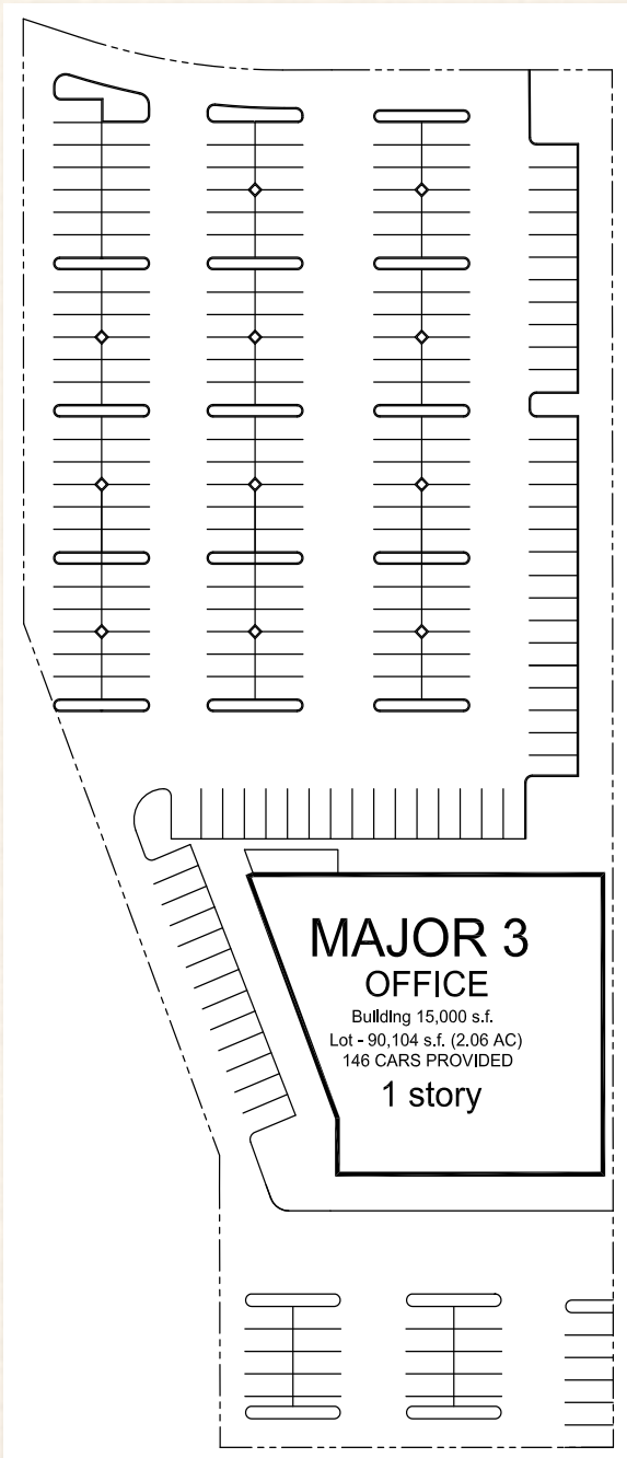
Siteplan
